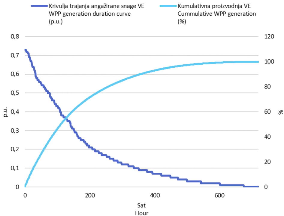
Slika 3 Krivulja trajanja angažirane snage svih VE i kumulativna proizvodnja VE u lipnju 2020. godine u jediničnim vrijednostima
