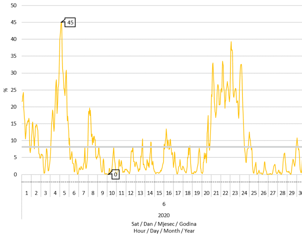
Slika 8 Udio proizvodnje vjetroelektrana u pokrivanju satnog opterećenja elektroenergetskog sustava u lipnju 2020. godine
