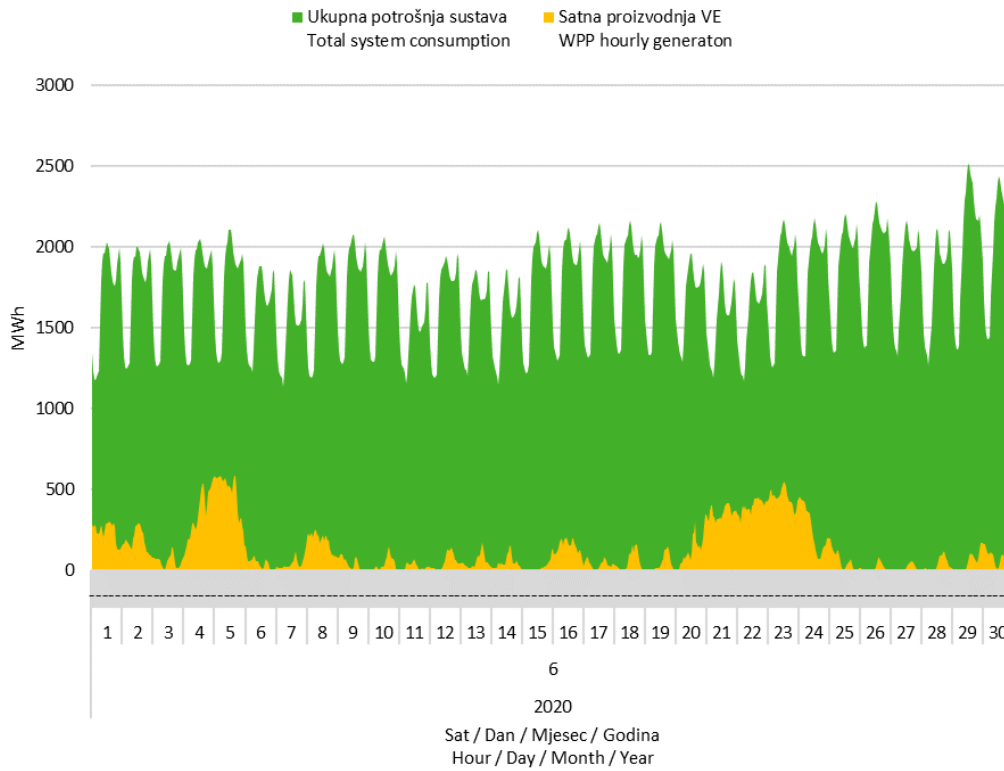
Slika 7 Usporedba satnog dijagrama opterećenja sustava i proizvodnje vjetroelektrana u lipnju 2020. godine
