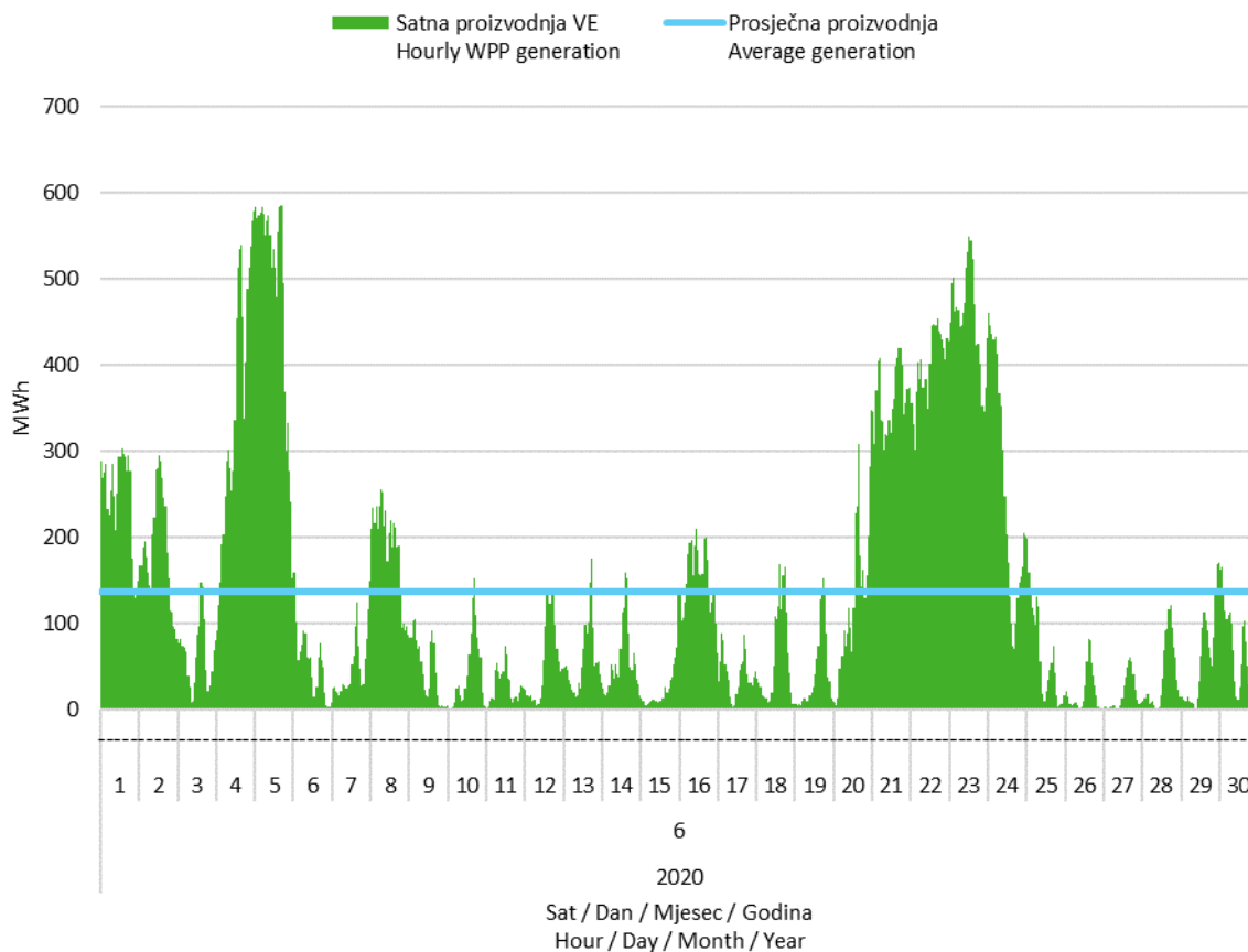
Slika 2 Satna proizvodnja svih vjetroelektrana u lipnju 2020. godine
