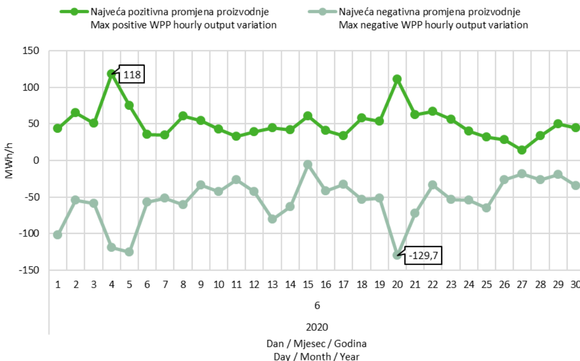
Slika 9 Maksimalna pozitivna i maksimalna negativna promjena satne proizvodnje VE u lipnju 2020. godine
