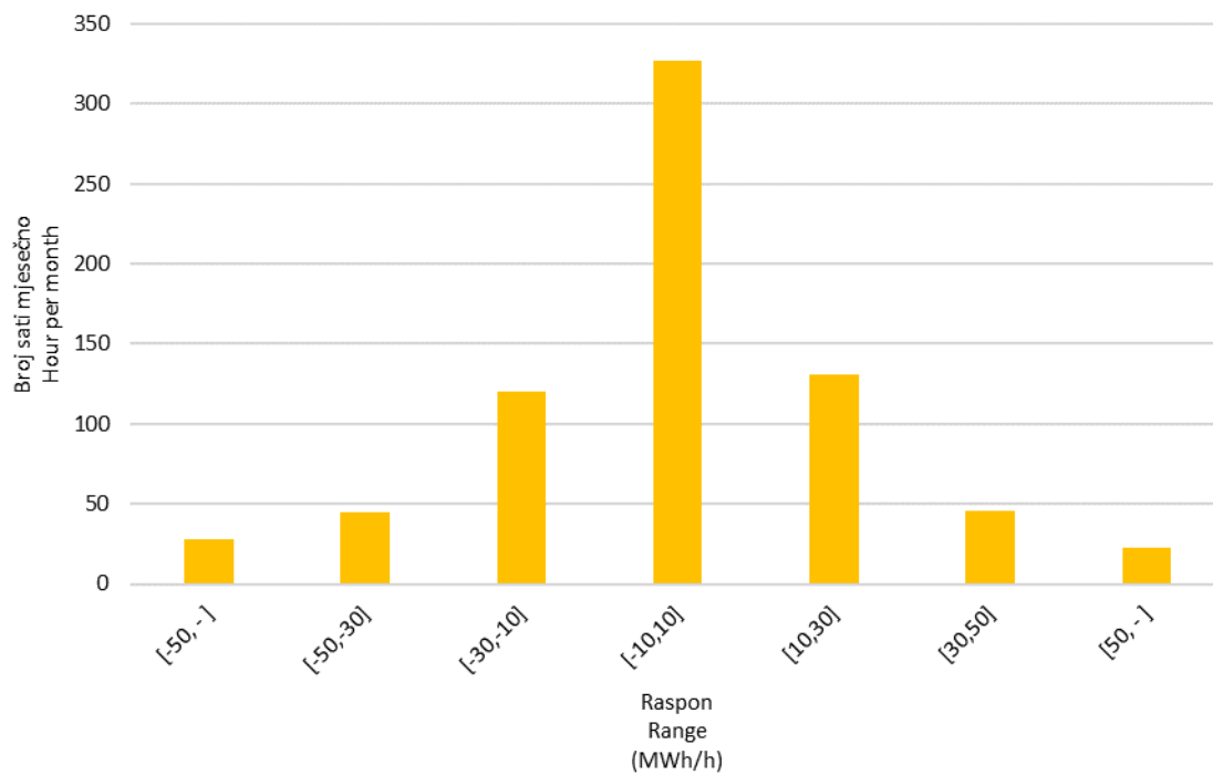
Slika 10 Statistička raspodjela satnih promjena proizvodnje VE u lipnju 2020. godine
