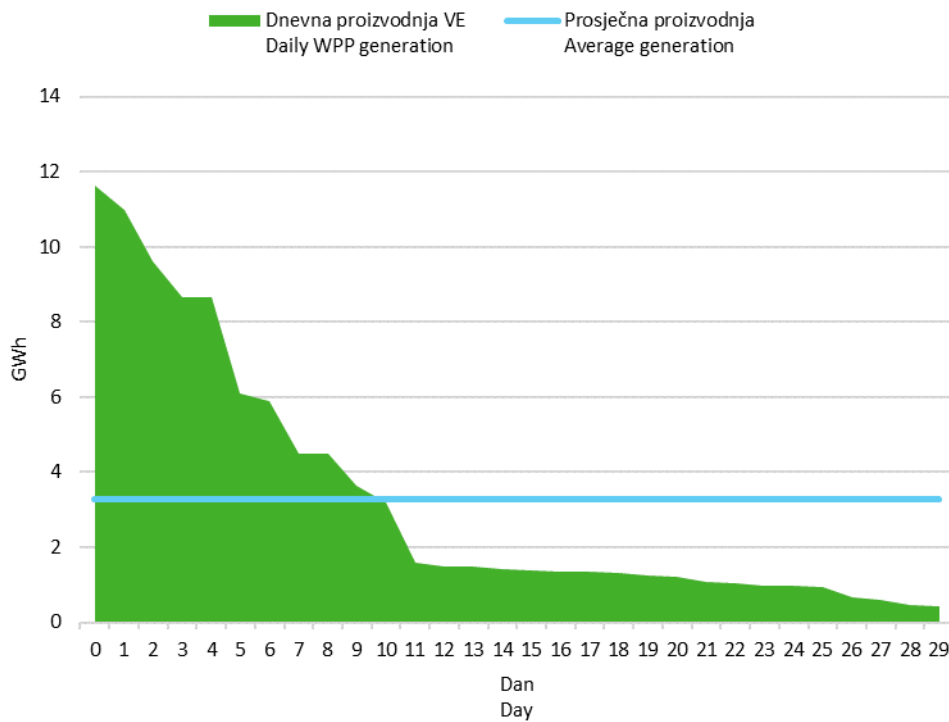
Slika 6 Krivulja trajanja dnevne proizvodnje vjetroelektrana u lipnju 2020. godine
