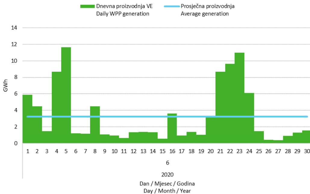
Slika 5 Dnevna proizvodnja svih vjetroelektrana u lipnju 2020. godine
